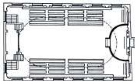
Ryc. 7. Plan Synagogi Schola Spagnola w Wenecji (XVI w). (wg C. H. Krinsky, 1985)
