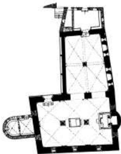
Ryc. 1. Plan synagogi w Wormacji (XI w.) Stan z poł. XIX w. (wg C. H. Krinsky, 1985)
